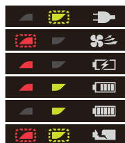
Ventilátor
